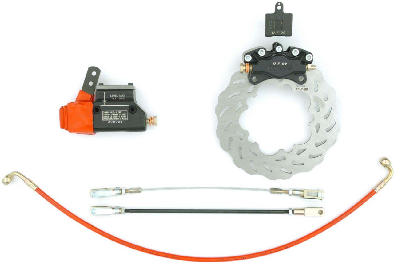
FOTO DEL SISTEMA FRENANTE COMPLETO
